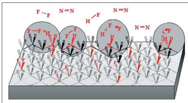
Im Idealfall bildet eine PTFE-Schicht – das heißt, alle oberflächlichen H-Atome sind durch F-Atome ersetzt – die Barrierschicht Foto: Air Products
